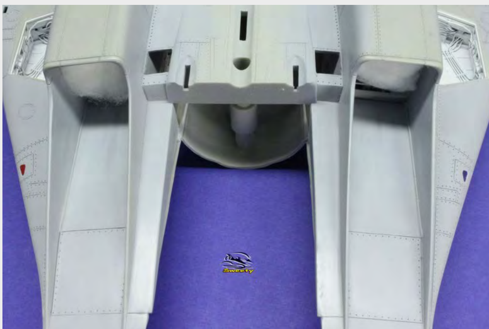
Mise en place de la crose d'appontage et préparation du logement des chaff and flare.
