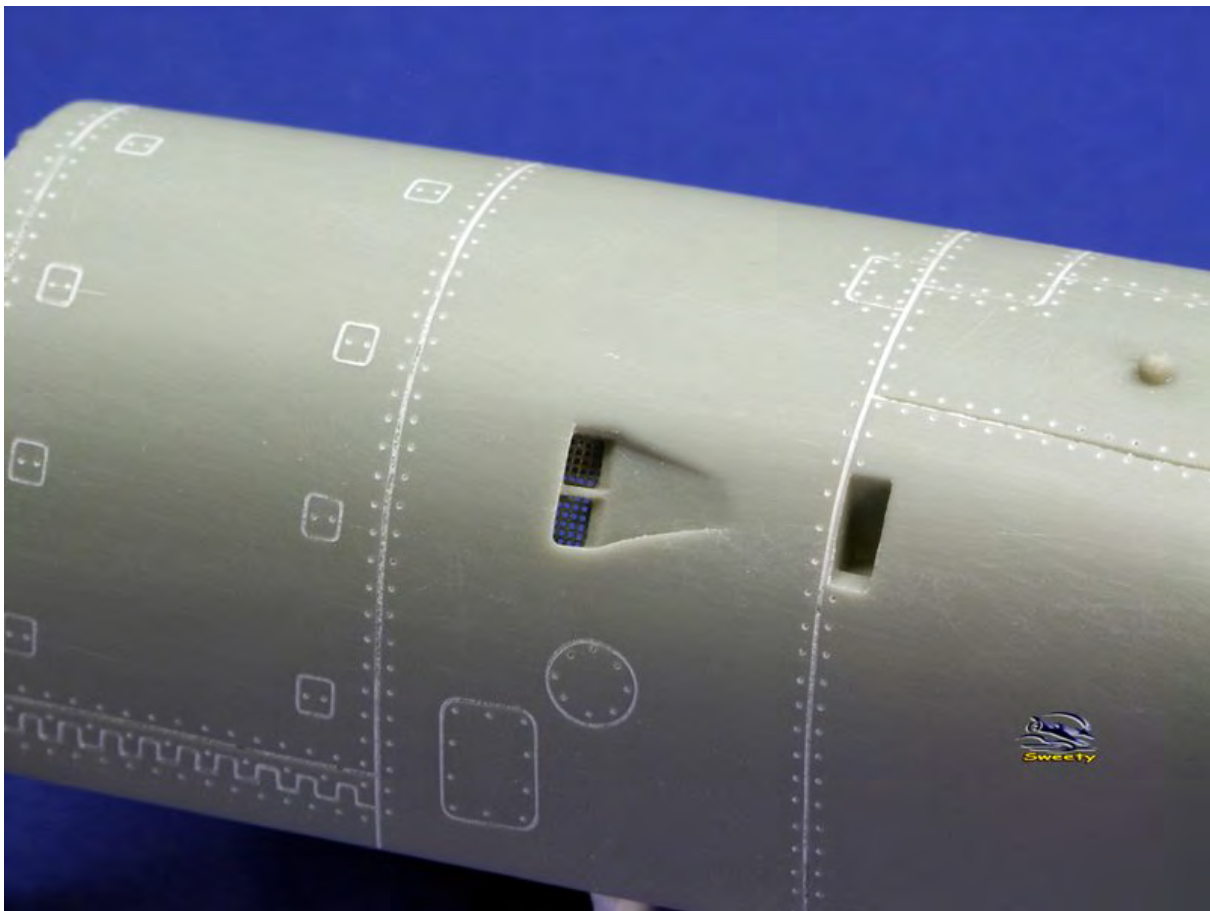
Maintenant je vais monter les volets de réglage du flux selon les vitesses subsoniques ou supersoniques. Je vais les monter en position subsonique c'est-à-dire fermées, pour cela il faut que je réalise un peu de photodec car il y a encore possibilité de voir l'intérieur du fuselage et surtout afin de voir le mécanisme d'ouverture. Photo ci-dessous.
